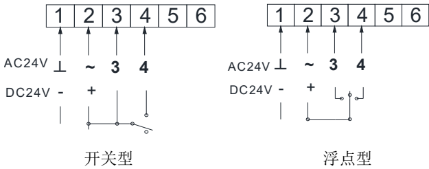
端子接线图
