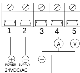
0~5V/0~10V/4~20mA(三线)
