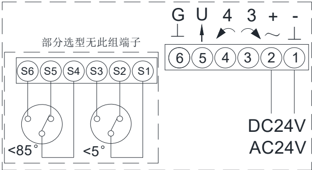
端子接线图
