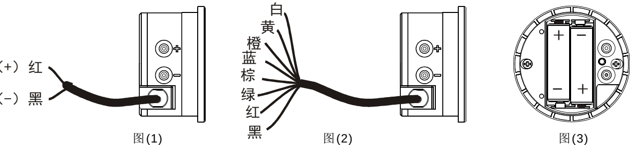
D5P/D5G/D5T 系列产品的 24VDC/AC 电源、继电器和变送器输出接线列表如下：
