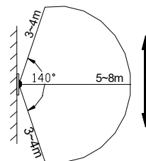
挂墙安装图示
