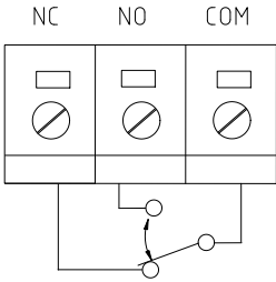
自动复位型(TCH-xA)接线图：
