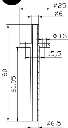
图 2: 连接件 1003
